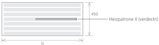
DRAUFSICHT
