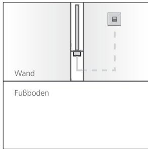
VORDERANSICHT
